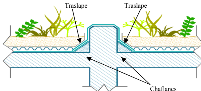
Figura 4. Impermeabilización en puntos de encuentro con elementos emergentes intermedios por debajo del nivel del substrato o de altura menor a 10cm sobre el nivel del mismo.
